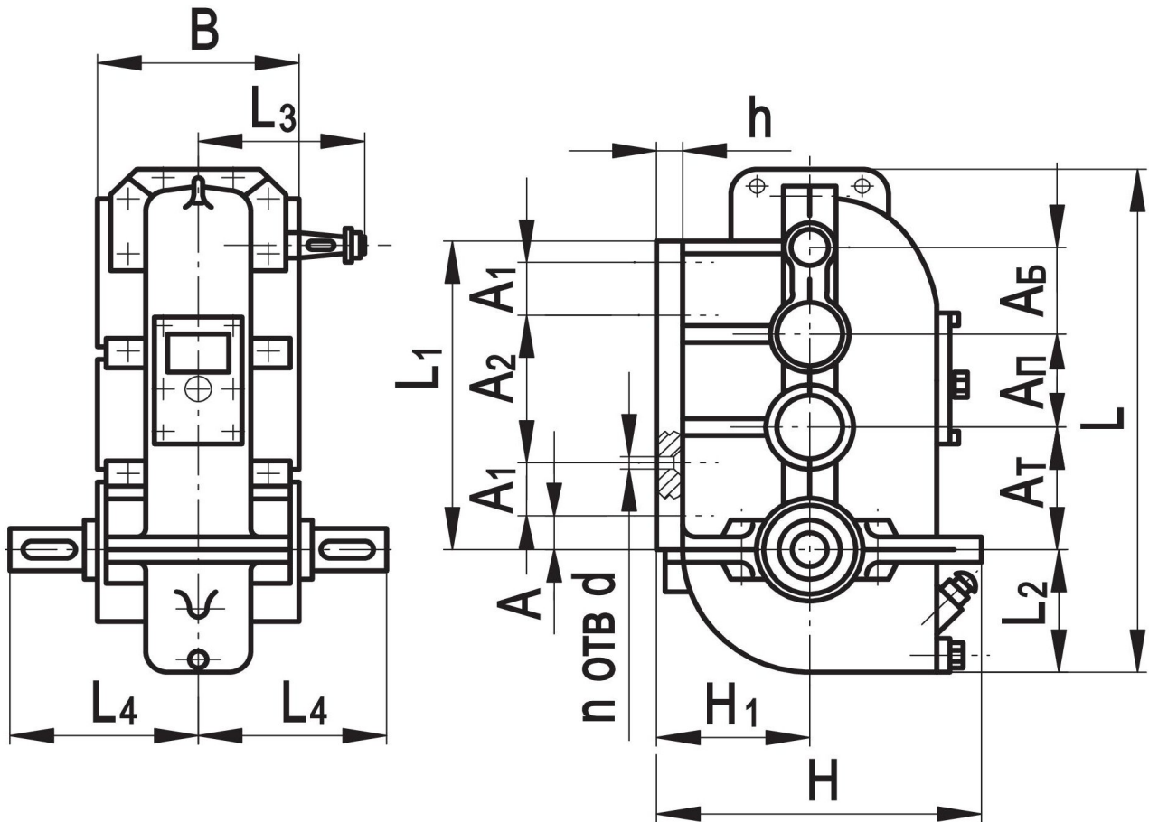
Редуктор ВК-550 Размеры и диаметр входного и выходного вала ВК-550
