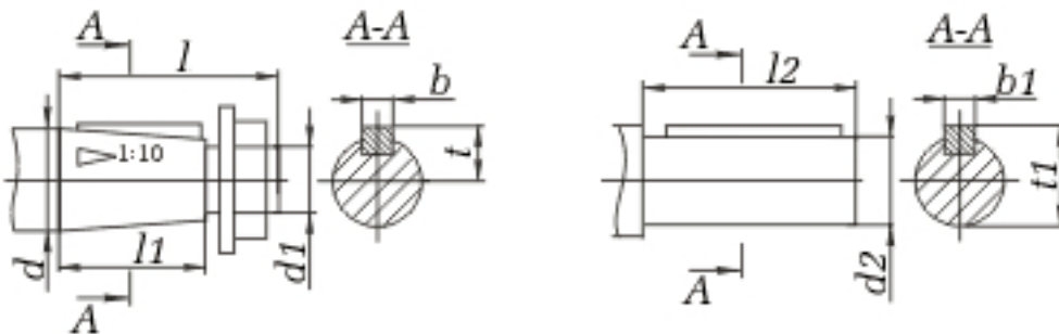
Редуктор ВК-550 Размеры и диаметр входного и выходного вала ВК-550
