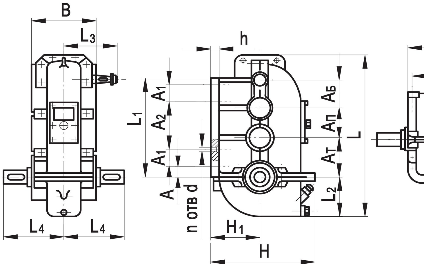
Редуктор ВК-475 Размеры и диаметр входного и выходного вала ВК-475 А Б 105 А П 60 А Т 210 ВХОДНОЙ
